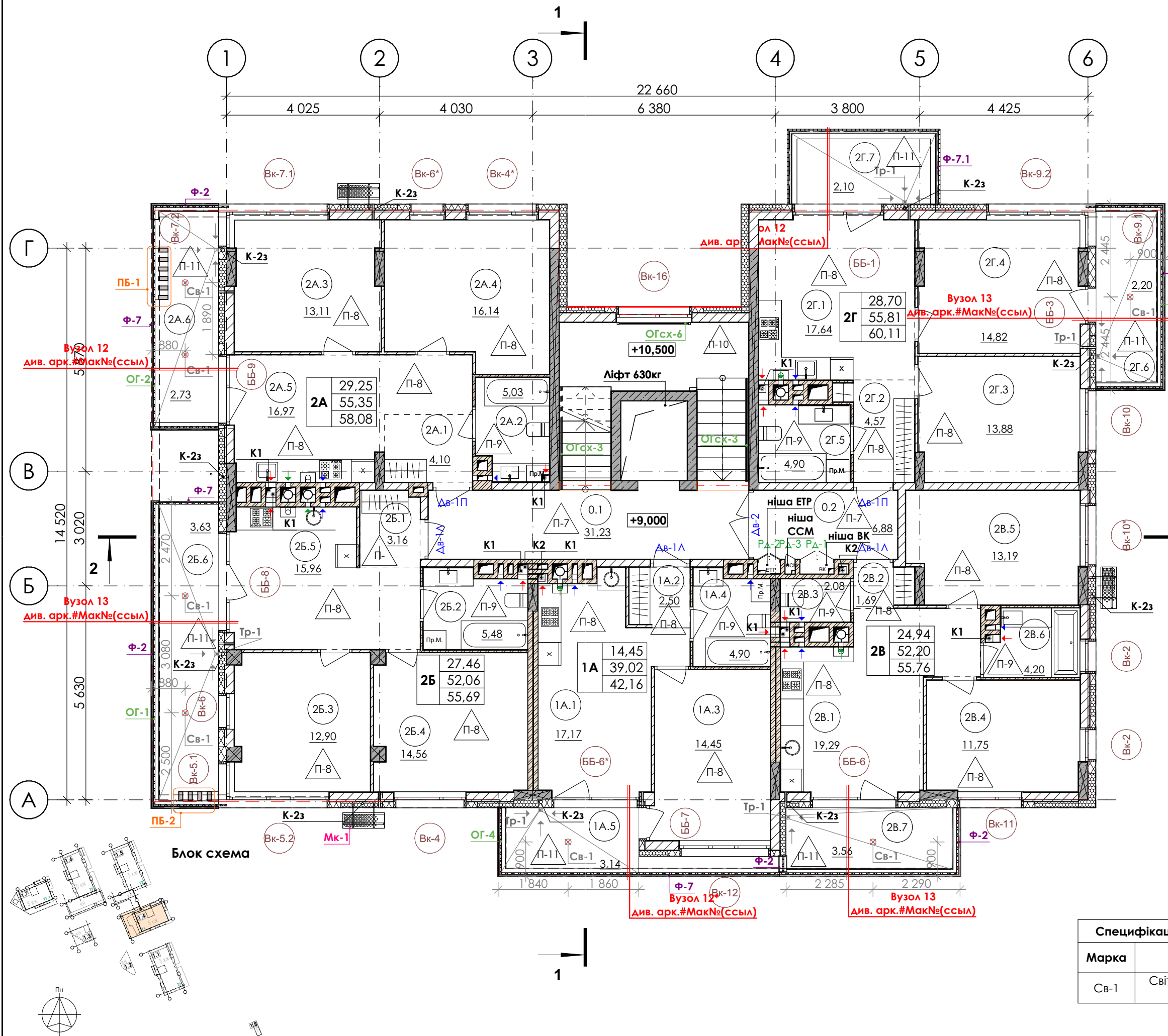
Маркувальний план 4 поверху на відм. +9,000 М 1:100
