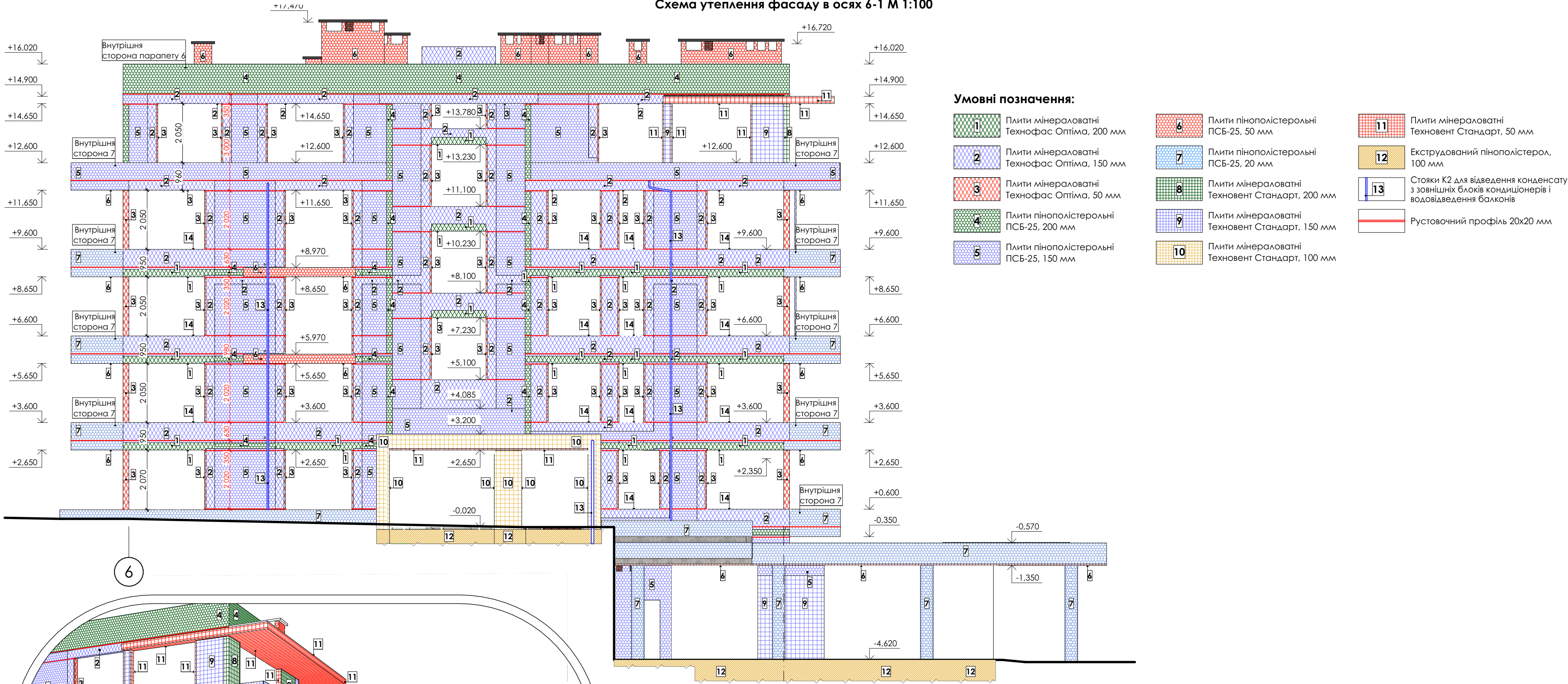
Схема утепления фасаду в осях 6-1 М 1:100
